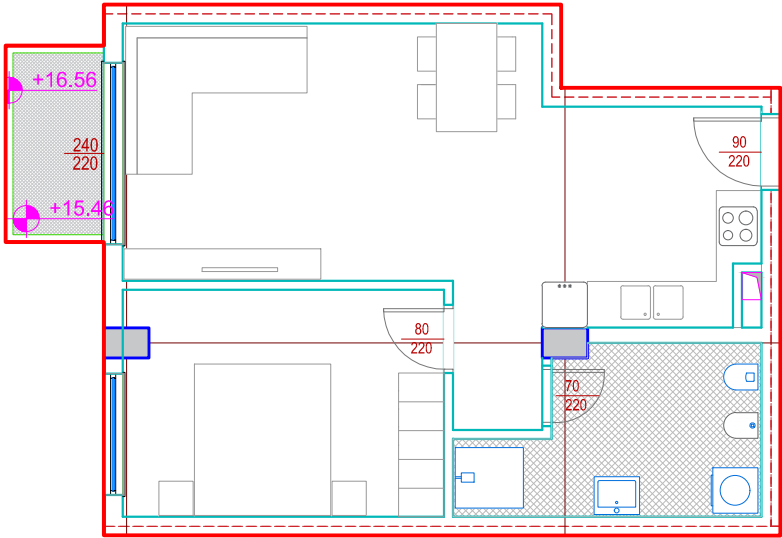
Planimetri Sh. 1:100 - Mobilimi -
