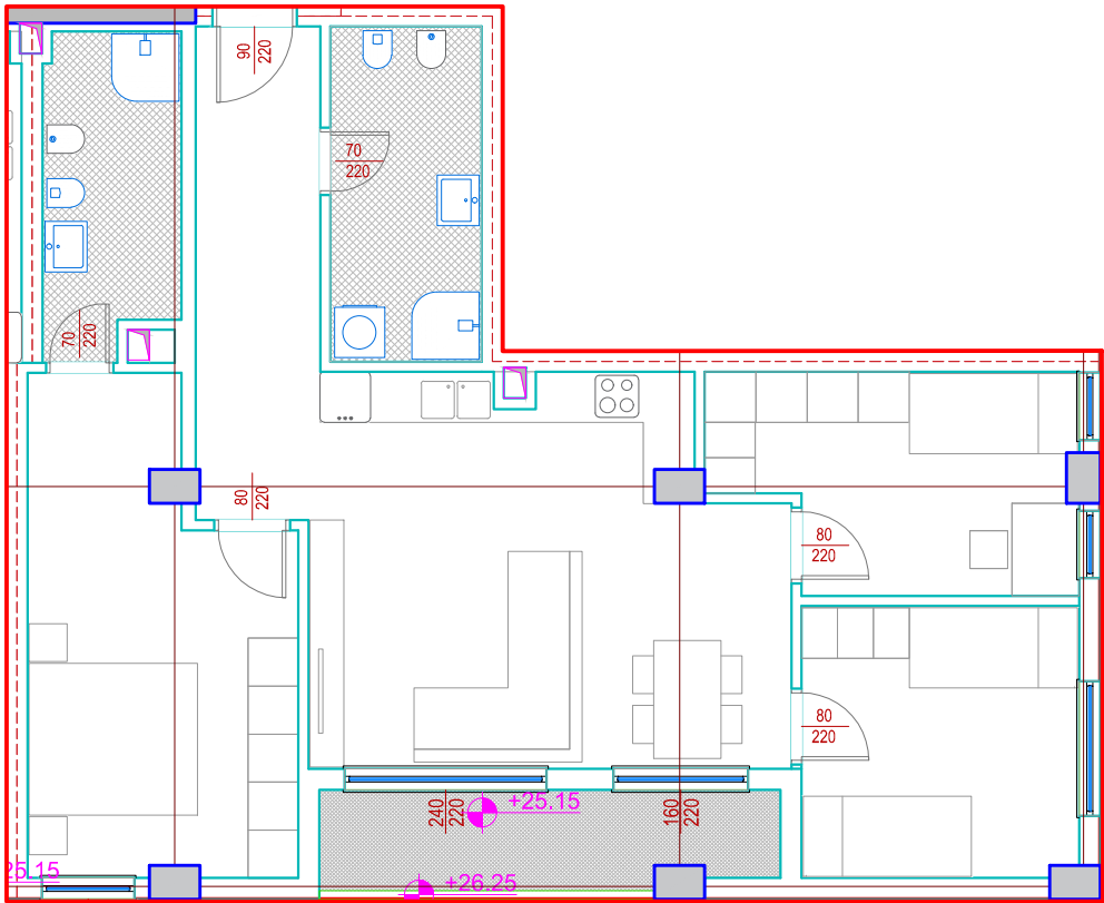
Planimetri Sh. 1:100 - Mobilimi -
