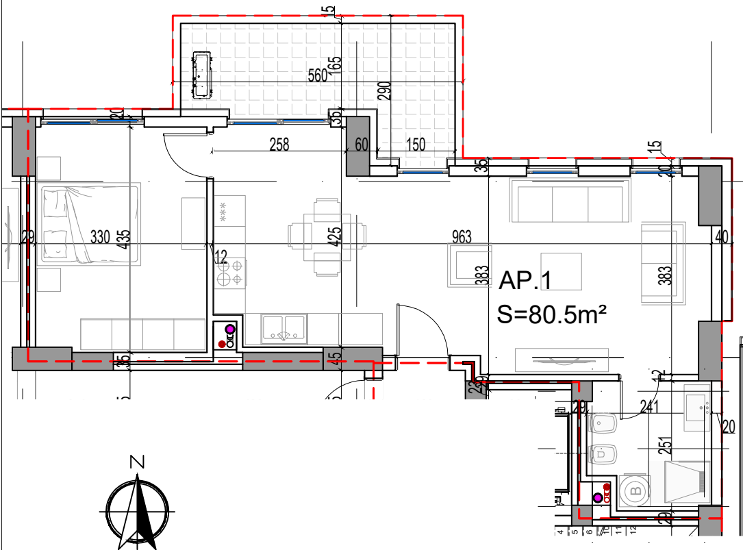
PLANIMETRIA E APARTAMENTIT SH 1:100 SEKSIONI B_KATI 1_SHKALLA 1_APARTAMENTI B-1_TIPI 1+1
