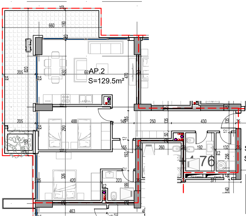
PLANIMETRIA E APARTAMENTIT SH 1:150 SEKSIONI B_KATI 1_SHKALLA 1_APARTAMENTI B-2_TIPI 2+1
