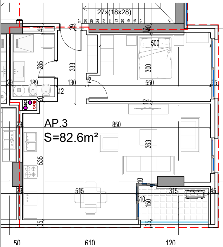
PLANIMETRIA E APARTAMENTIT SH 1:100 SEKSIONI B_KATI 1_SHKALLA 2_APARTAMENTI B-3_TIPI 1+1
