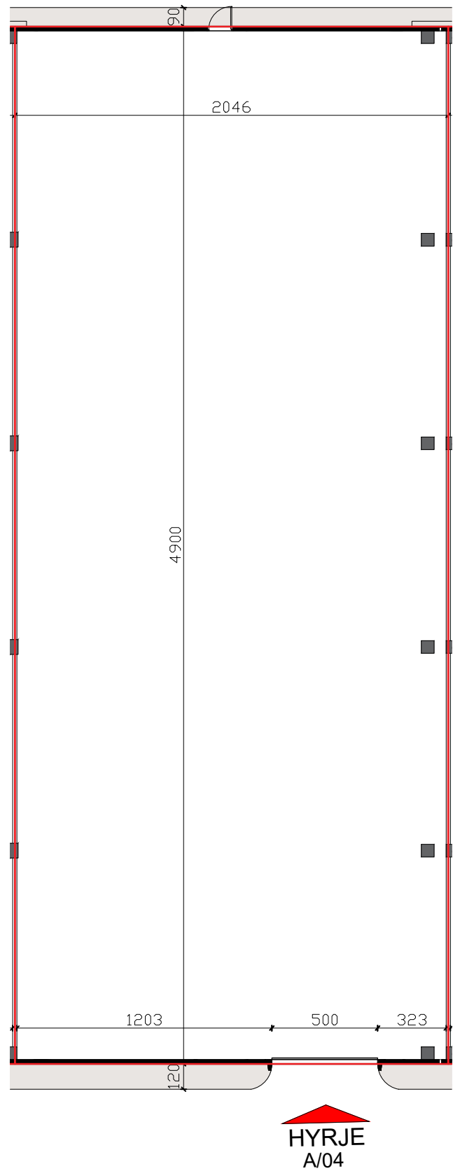
PLANIMETRIA E NJËSISË SHKALLA 1 : 250
