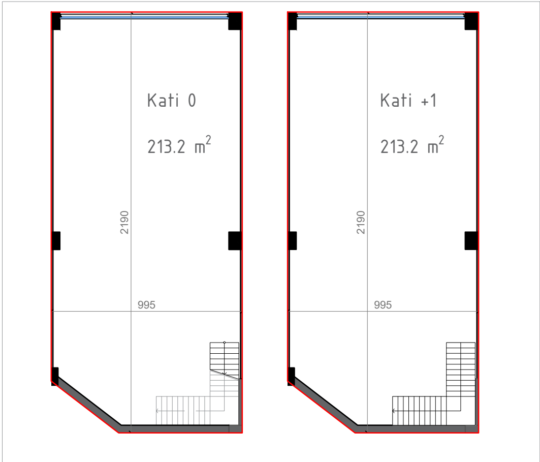
PLANIMETRITË E NJËSISË : Kati 0 & Kati 1
